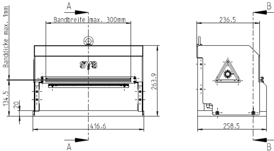
Zeichnung BDML-300
